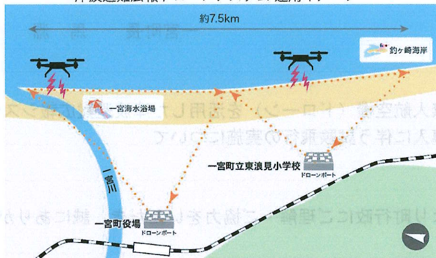
津波避難広報ドローンシステム 運行ルート
