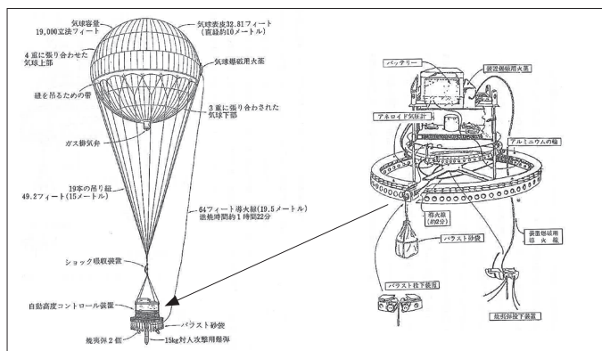
▲風船爆弾の構造 (木下健蔵『消された秘密戦研究所』(信濃毎日新聞社、1994年)掲載図より引用)
